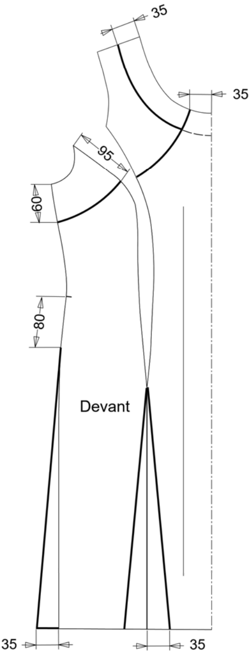
PLAN DE COUPE
